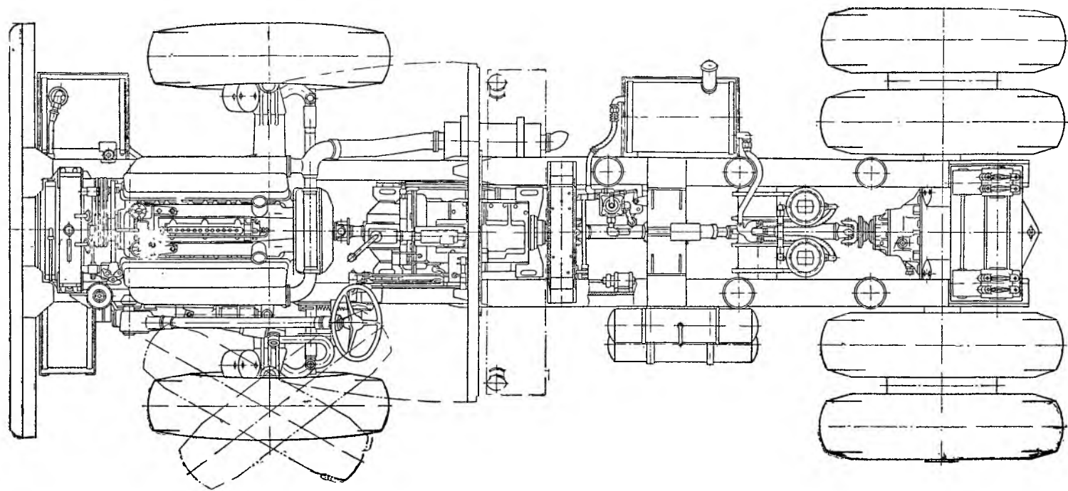
Фиг. 4. Шасси автомобиля-самосвала МАЗ-525
