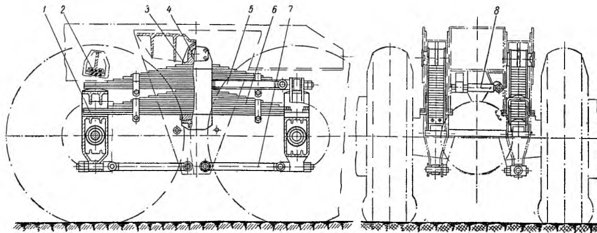
Фиг. 71. Задняя подвеска автомобиля МАЗ-530:
