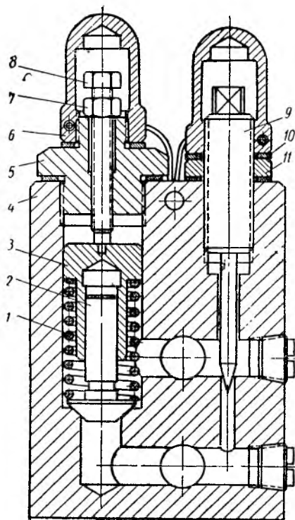
Фиг. 76. Регулятор скорости и давления:
