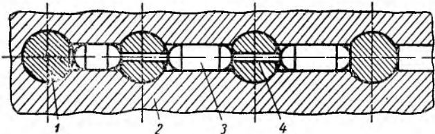
Фиг. 40. Блокирующее устройство механизма переключения передач: 1 — шток, 2 — верхняя крышка коробки; 3 — сухарь, 4 — штифт
