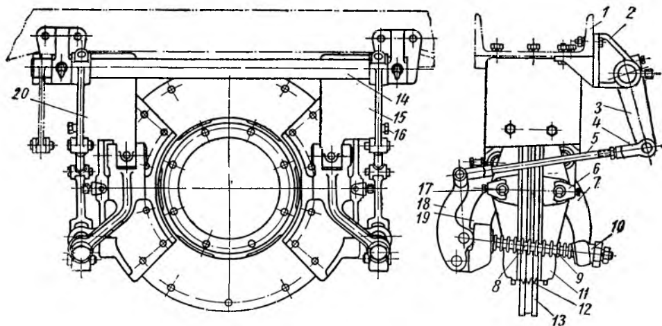
Фиг. 91. Ручной тормоз автомобиля МАЗ-525:
