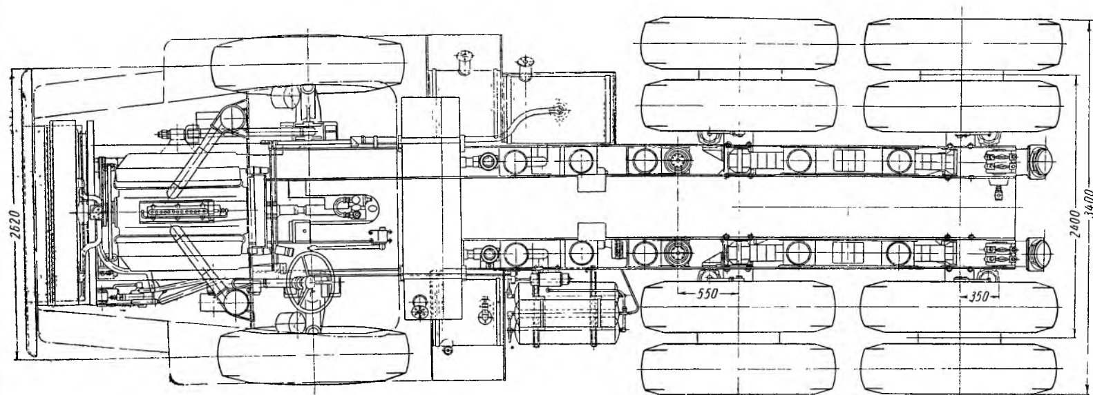
Фиг. 5. Шасси автомобиля-самосвала МАЗ-530.
