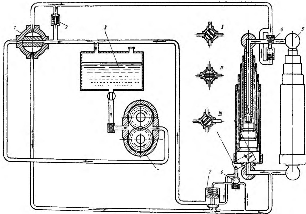
Фиг. 109. Схема гидравлического оборудования опрокидывающего механизма: 1 — кран управления; 2 — предохранительный клапан принудительного опускания платформы; 3 — масляный бак; 4 — дроссельный клапан; 5 — цилиндр; 6 — датчик; 7 — сливной клапан; 8 — насос.
