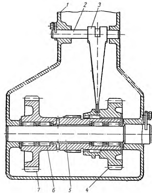
Фиг. 39. Ось шестерен заднего хода: 1 — картер коробки передач; 2 — ось вилок; 3 — подвижная вилка заднего хода; 4 — каретка; 5 — ось шестерен; 6 — радиальный роликоподшипник; 7 — шестерня заднего хода.
