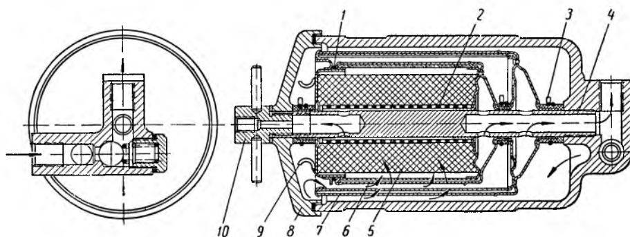
Фиг. 28. Масляный фильтр:
