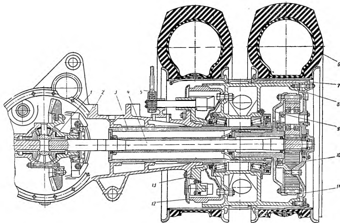
Фиг. 65. Средний и задний ведущие мосты автомобиля МАЗ-530:
