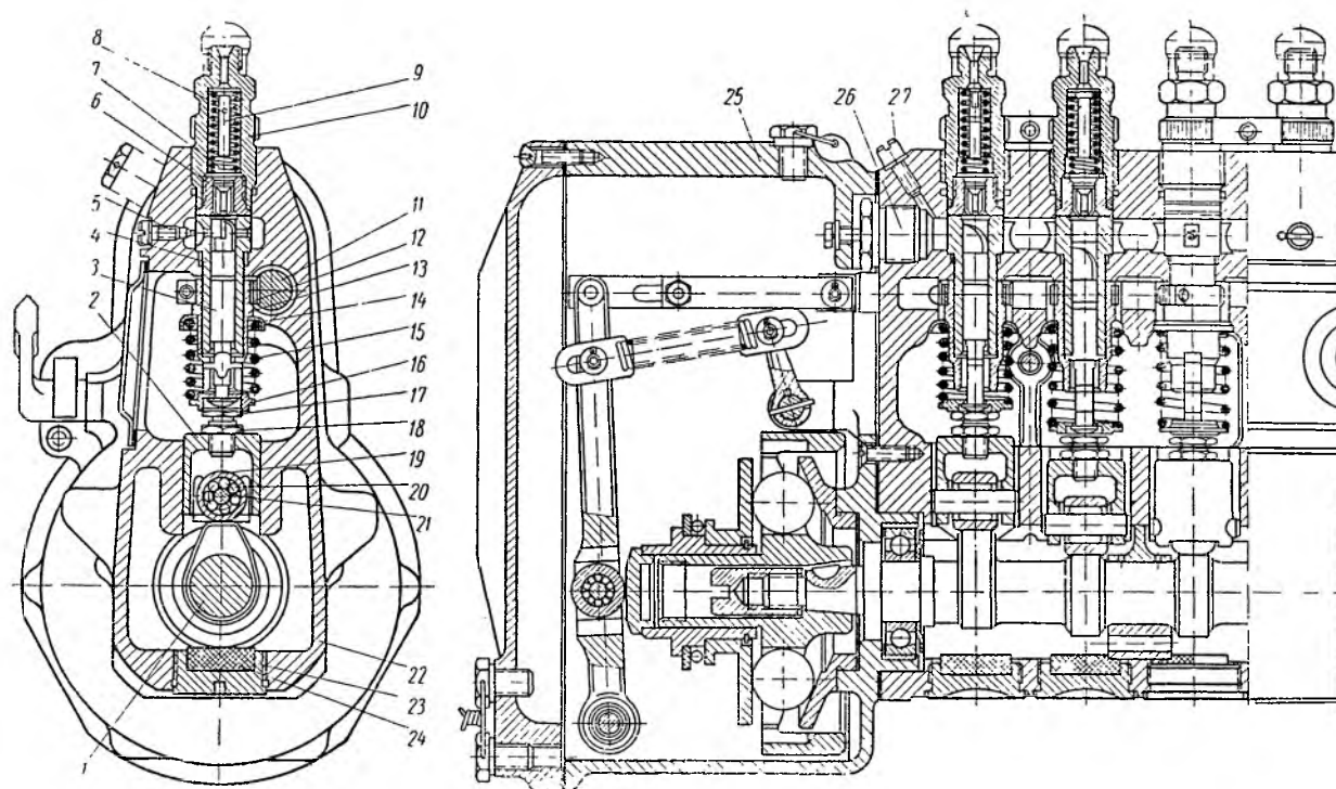
Фиг. 22. Топливный насос:
