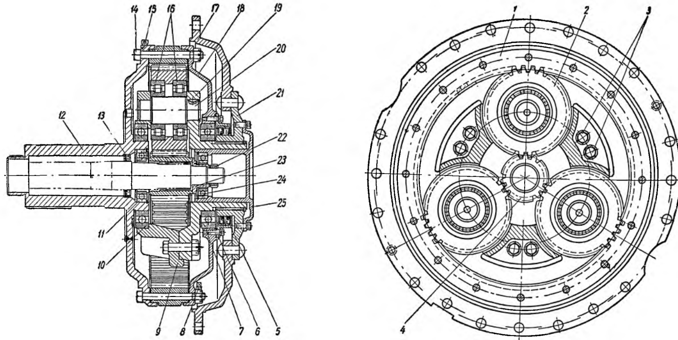
Фиг. 62. Планетарный редуктор автомобиля МАЗ-525:
