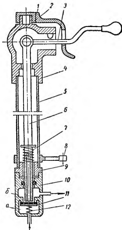
Фиг. 52. Схема установки рычага переключения передач и клапана включения заднего хода:
