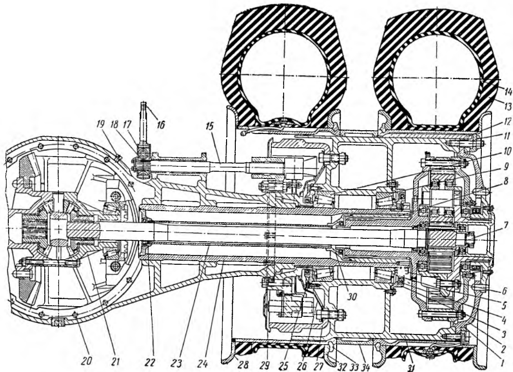
Фиг. 64. Задний мост автомобиля МАЗ-525: 1 — направляющий диск клиньев; 2 — планетарный редуктор; 3 — наружная крышка ступицы; 4 — сальник; 5 — гайка подшипника; 6 — контргайка; 7 — полуось; 8 — муфта; 9 — наружный подшипник; 10 — внутренний подшипник; 11 — прижим; 12 — клин крепления колеса; 13 — покрывка; 14 — камера; 15 — разжимной кулак заднего тормоза; 16 — регулировочный рычаг; 17 — червяк регулировочного рычага; 18 — шестерня регулировочного рычага; 19 — тапун; 20 — картер заднего моста; 21 — дифференциал; 22 — корпус сальника полуоси; 23 — труба полуоси; 24 — кожух полуоси; 25 — внутренняя крышка ступицы; 26 — маслоотражатель; 27 — тормозной барабан; 28 — обод колеса; 29 — защитный диск; 30 — фланец трубы; 31 — ступица; 32 — бортовое кольцо; 33 — замочное кольцо; 34 — распорное кольцо.
