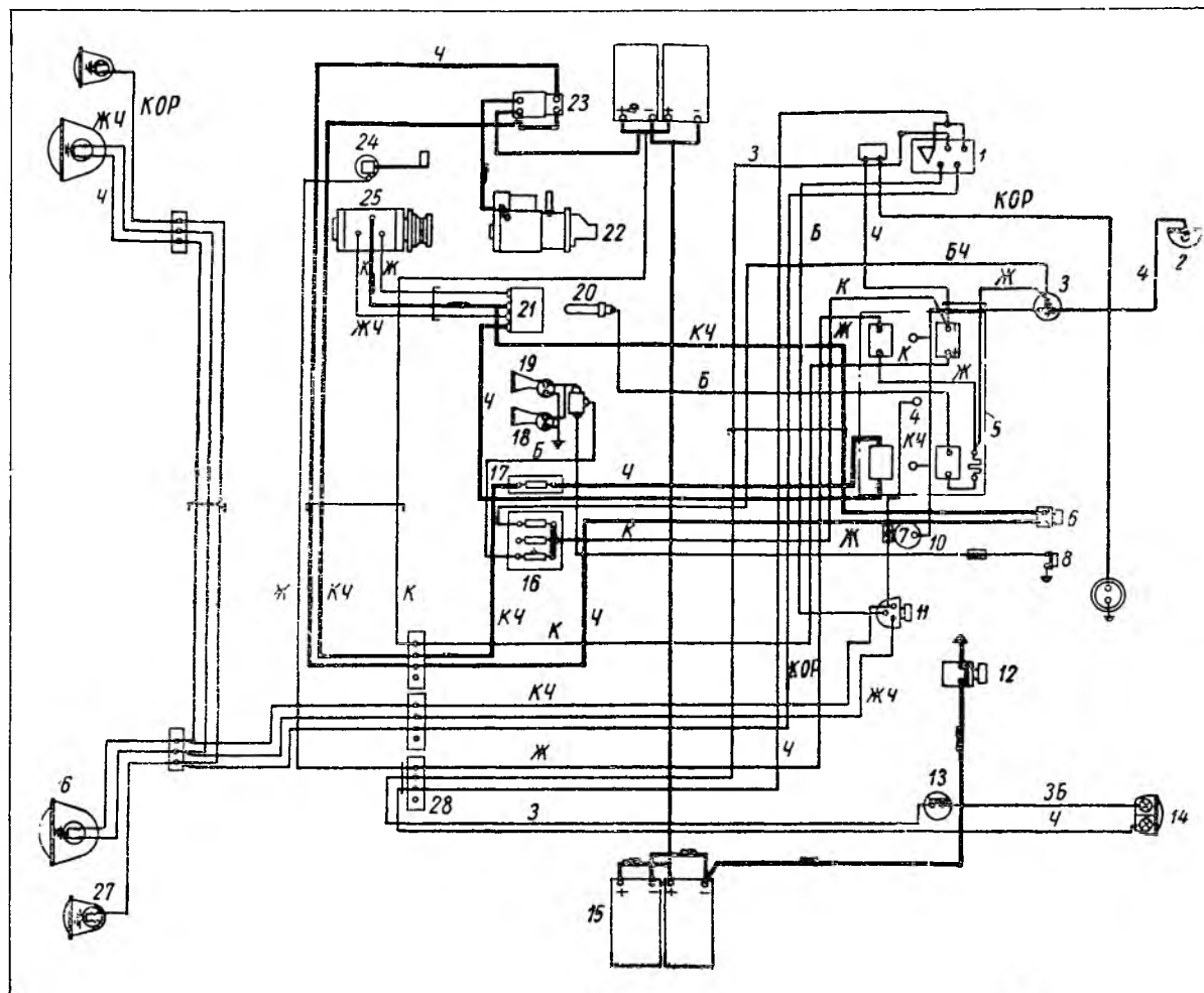
Фиг. 93. Принципиальная схема электрооборудования автомобиля МАЗ-525:
