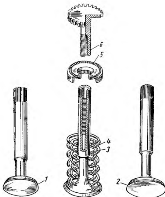
Фиг. 16. Клапаны: 1 — выпускной клапан; 2 — впускной клапан; 3 — внутренняя пружина; 4 — наружная пружина; 5 — замок головки клапана; 6 — головка клапана.
