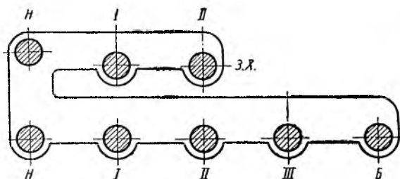
Фиг. 51. Схема положений рычага переключения передач (развертка ограничителя рычага по направляющим пазам).
