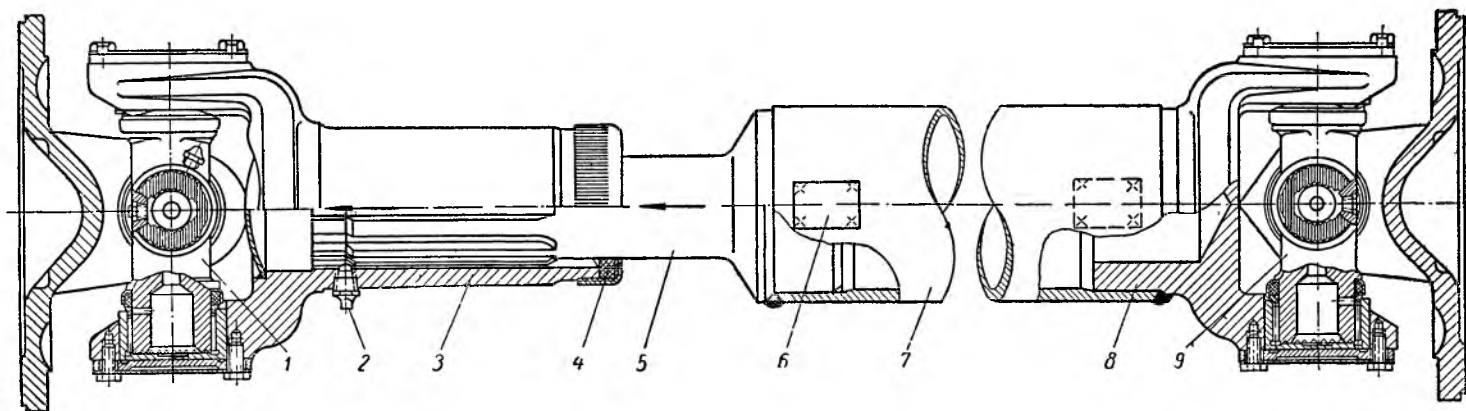
Фиг. 57. Карданный вал автомобиля МАЗ-525:
