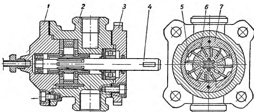
Фиг. 77 Насос гидравлического усилителя рулевого управления автомобиля МАЗ-525:
