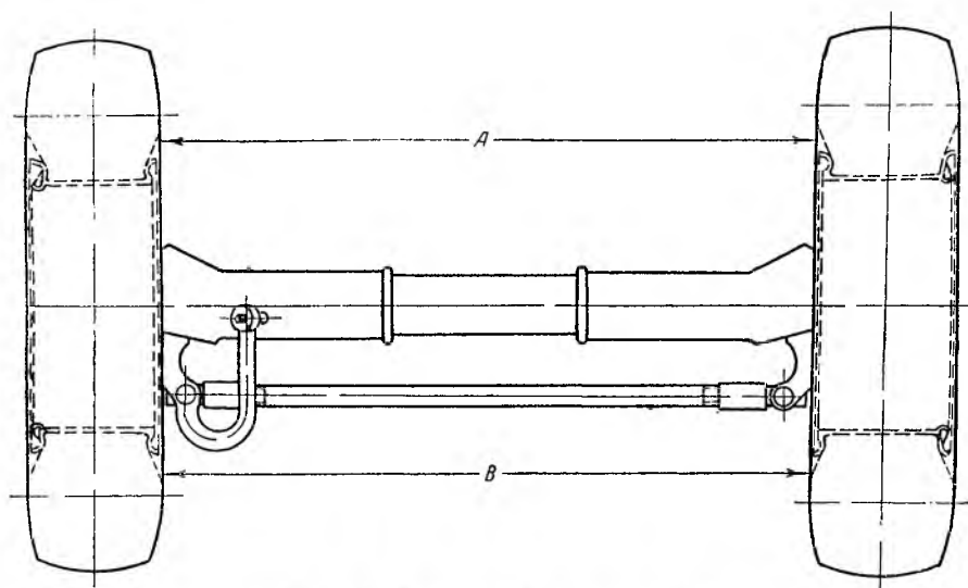
Фиг. 68. Схождение передних колес.
