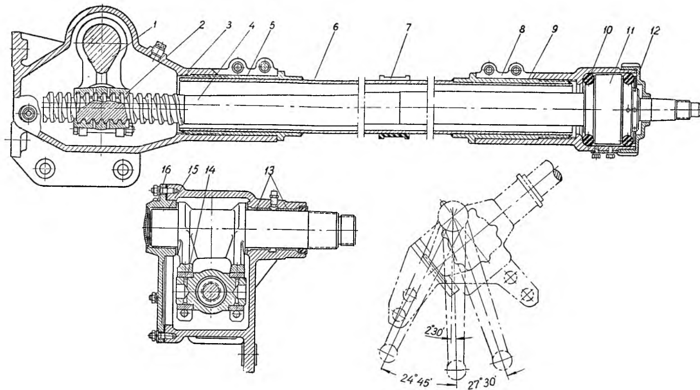
Фиг. 73. Рулевой механизм:
