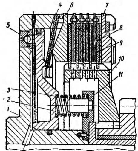
Фиг. 45. Фрикцион коробки передач:
