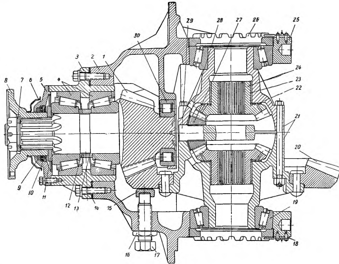
Фиг. 61. Редуктор заднего моста автомобиля МАЗ-525:
