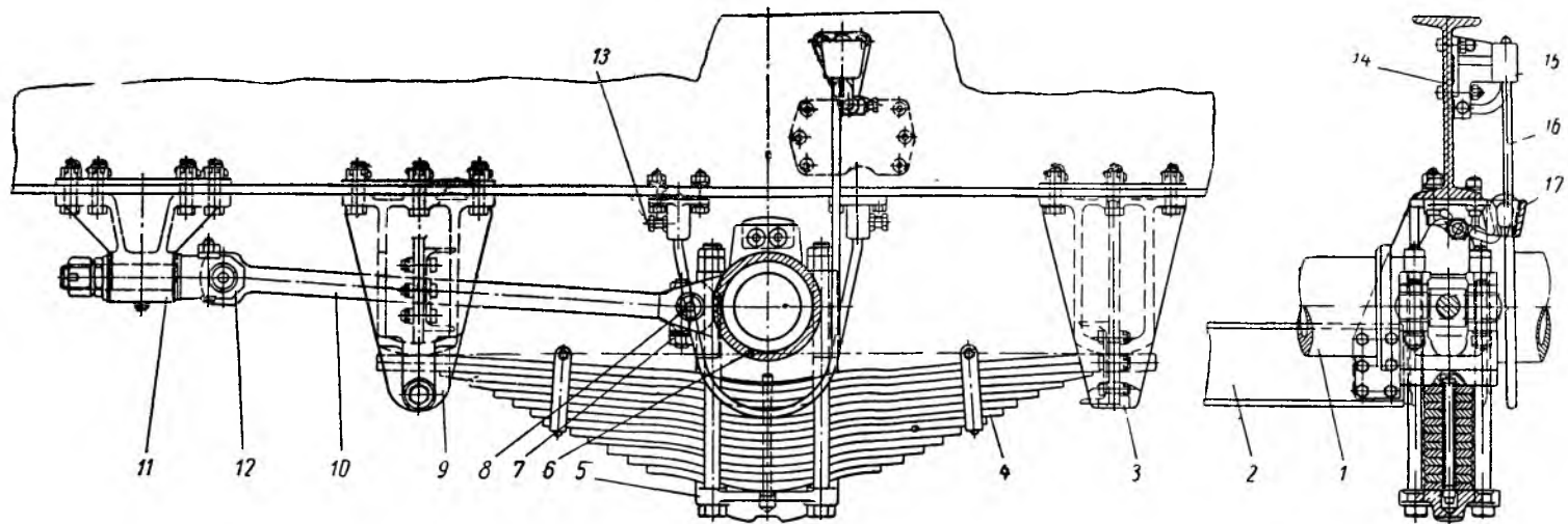
Фиг. 69. Передняя подвеска автомобиля МАЗ-525:
