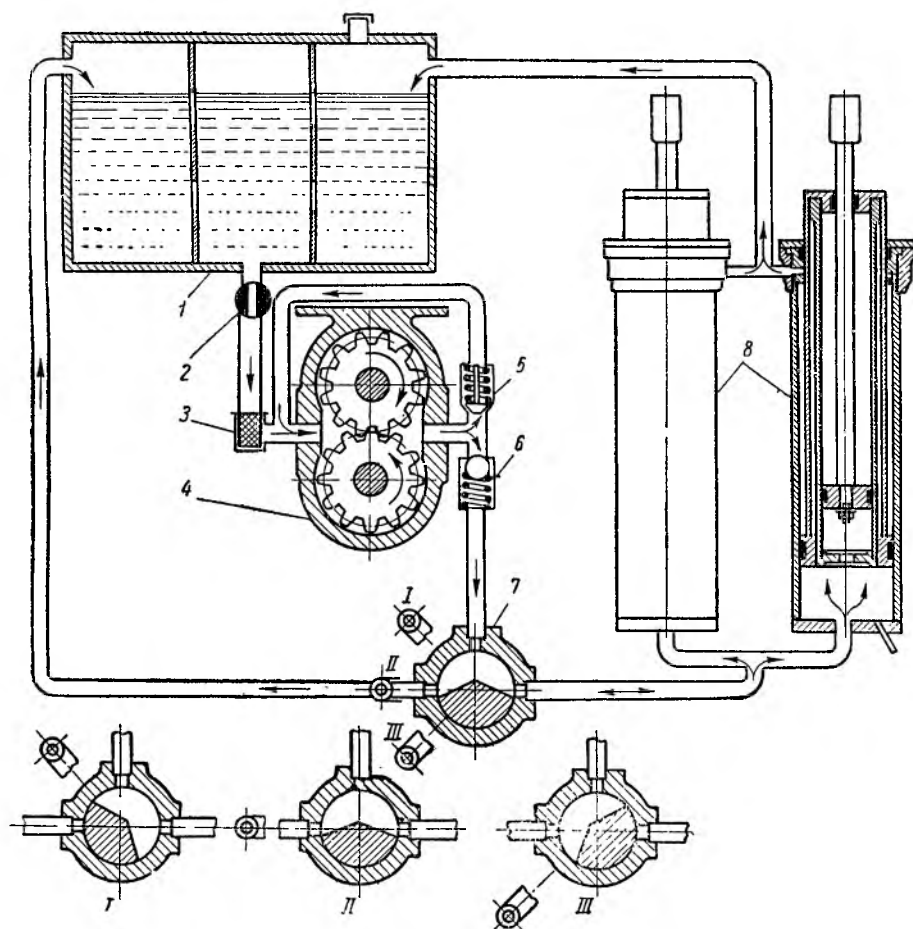
Фиг. 103. Схема гидравлического оборудования опрокидывающего механизма: 1 — масляный бак; 2 — переключательный кран; 3 — фильтр; 4 — насос; 5 — предохранительный клапан; 6 — обратный клапан; 7 — кран управления; 8 — цилиндры.
