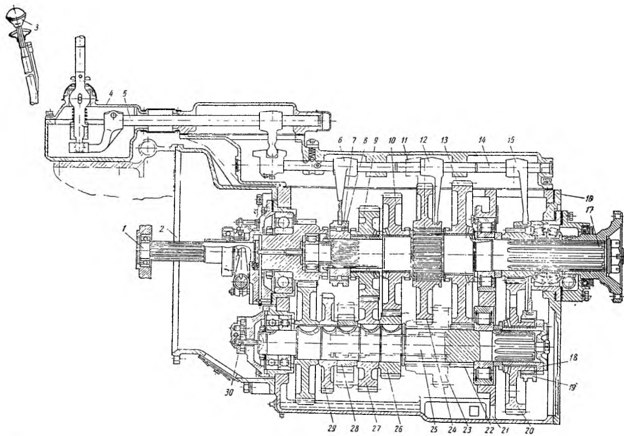
Фиг 38. Коробка передач автомобиля МАЗ-525:
