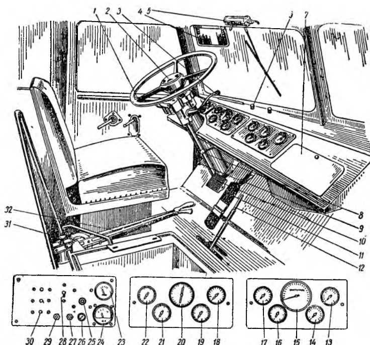
Фиг. 7. Органы управления и контрольно-измерительные приборы автомобиля МАЗ-530:
