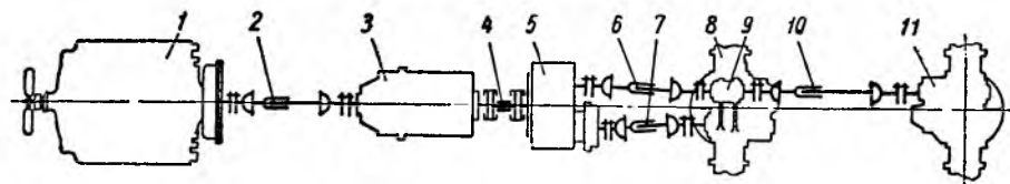
Фиг. 56. Схема установки карданных валов автомобиля МАЗ-530:
