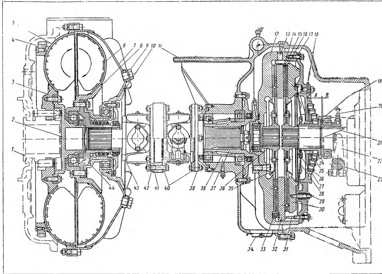
Фиг. 35 Гидрсмфта и сцепление:
